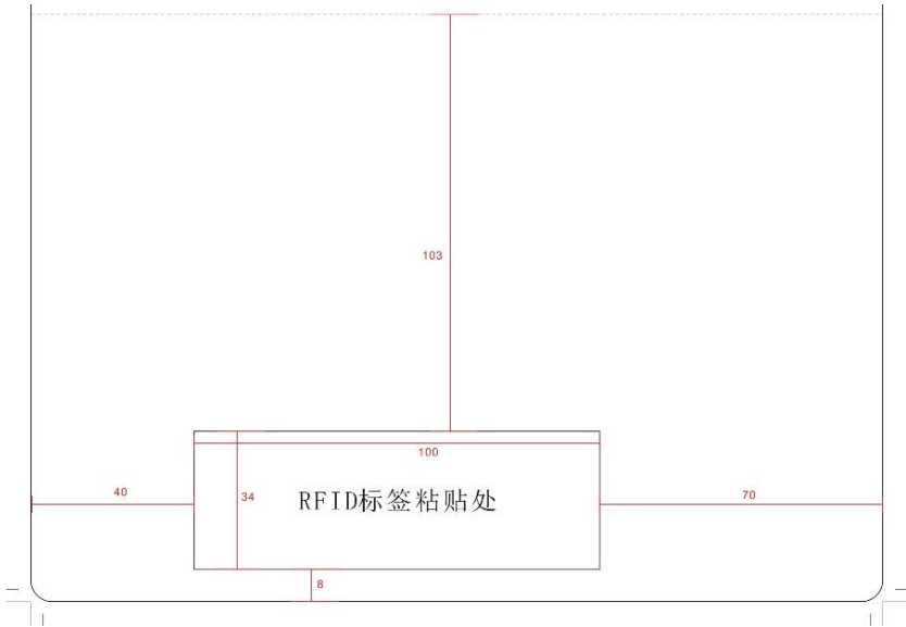
图 1-2-10 RFID 标签粘贴示意图
