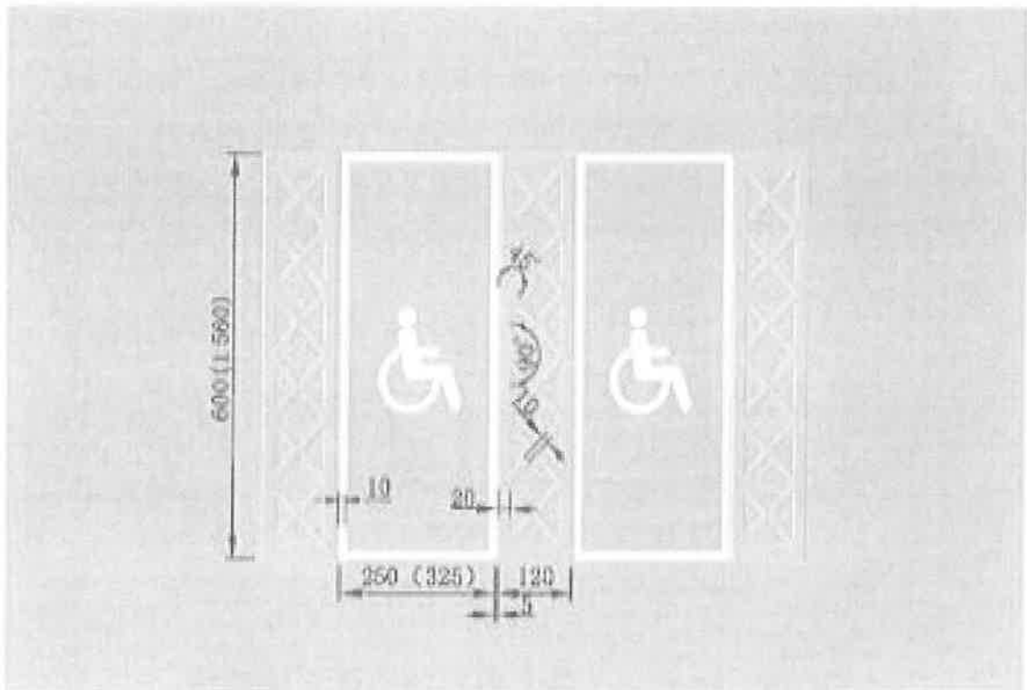
图 31 线 25 残疾人专用停车位标线
