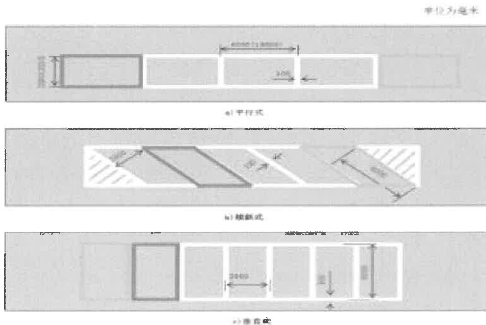
图1 停车泊位排列形式
