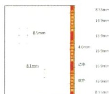
图 A.2 热敏涂层面图案 B
