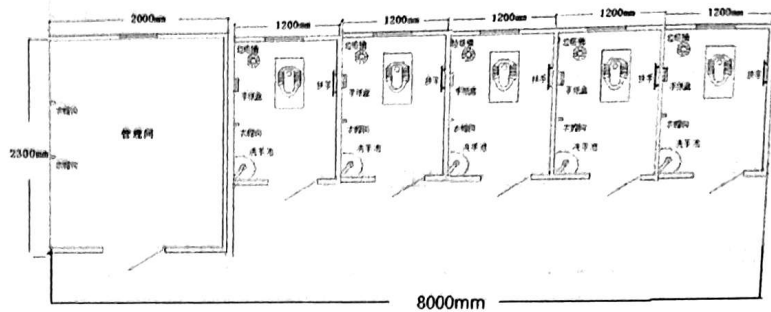
厕所平面布局图
