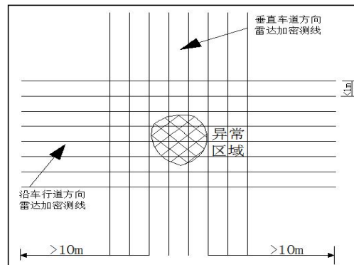
异常区域复测测线布置示意图
