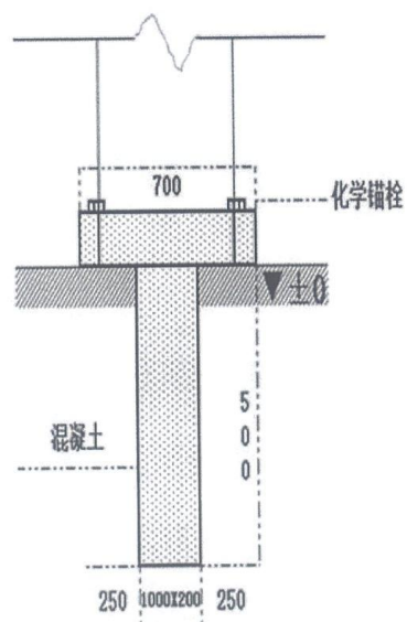
剖面图
