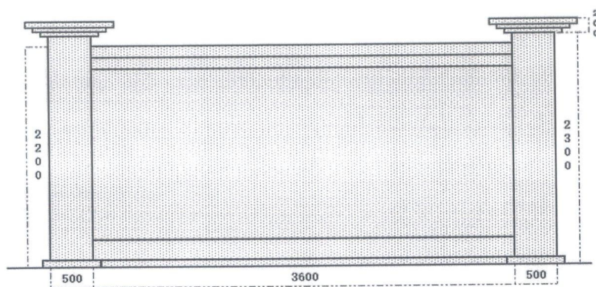
产品结构正面图
