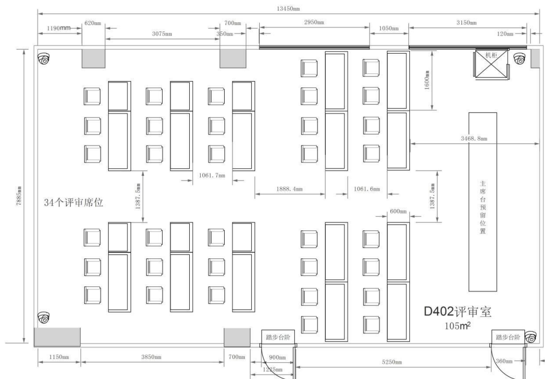
图 1 平面布局图
