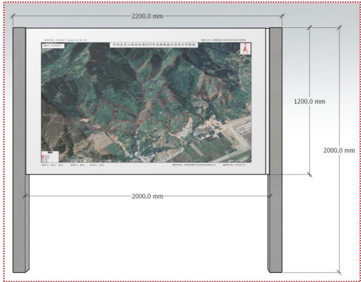
简介牌规格制作图
