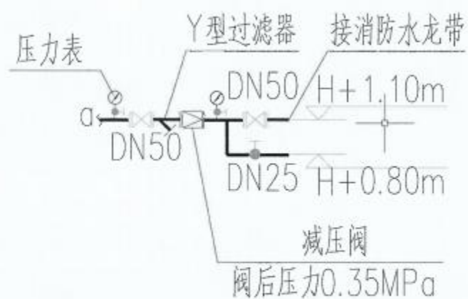
管道连接大样图 a
