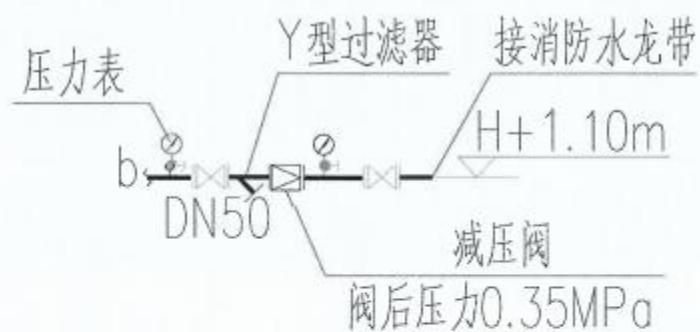
管道连接大样图 b
