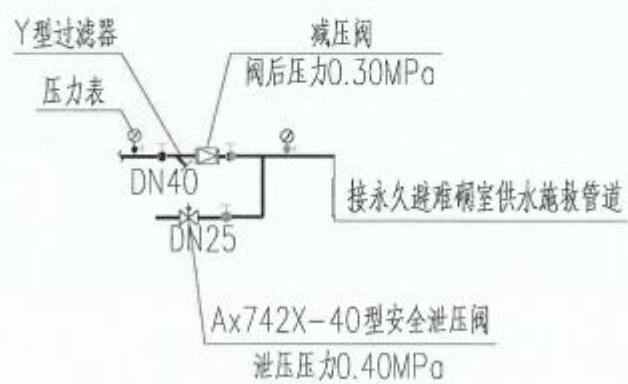
永久避难硐室减压阀安装大样
