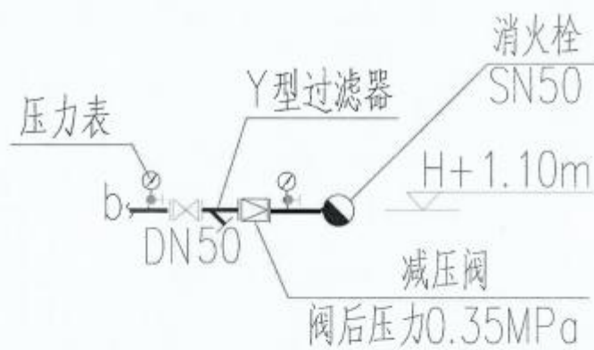
消火栓节点大样图
