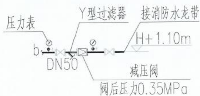
管道连接大样图 b
