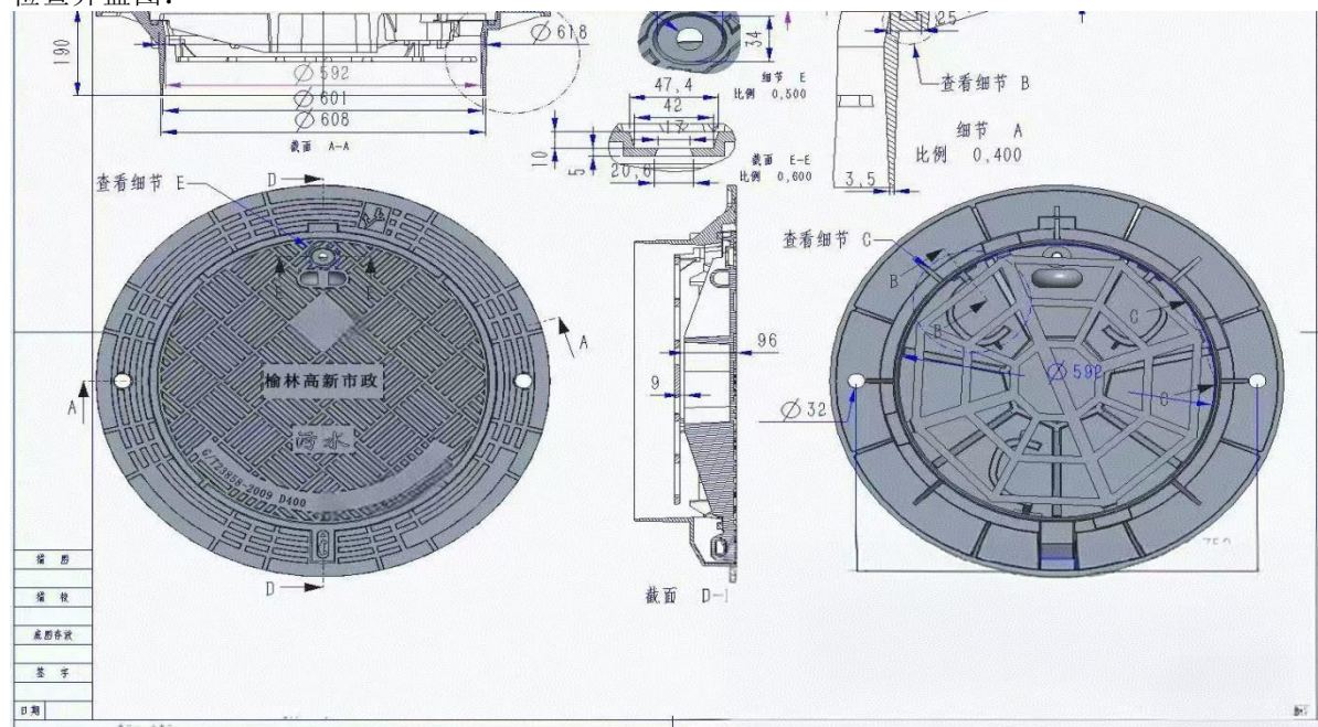
检查井盖图:
