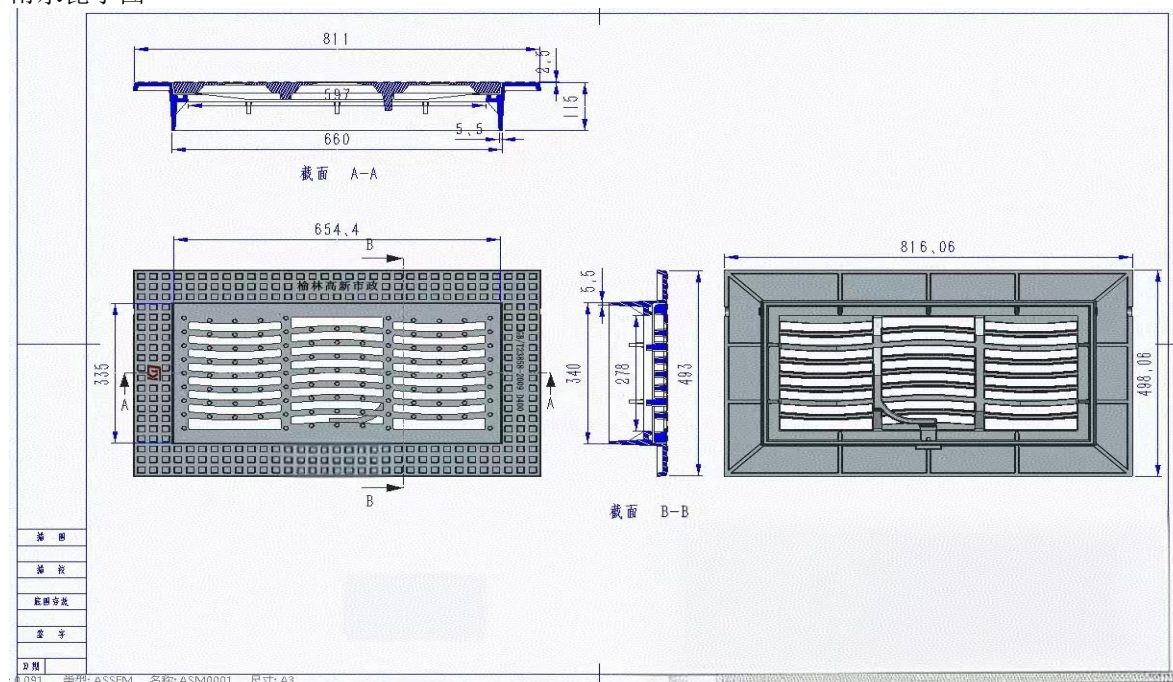
雨水篦子图
