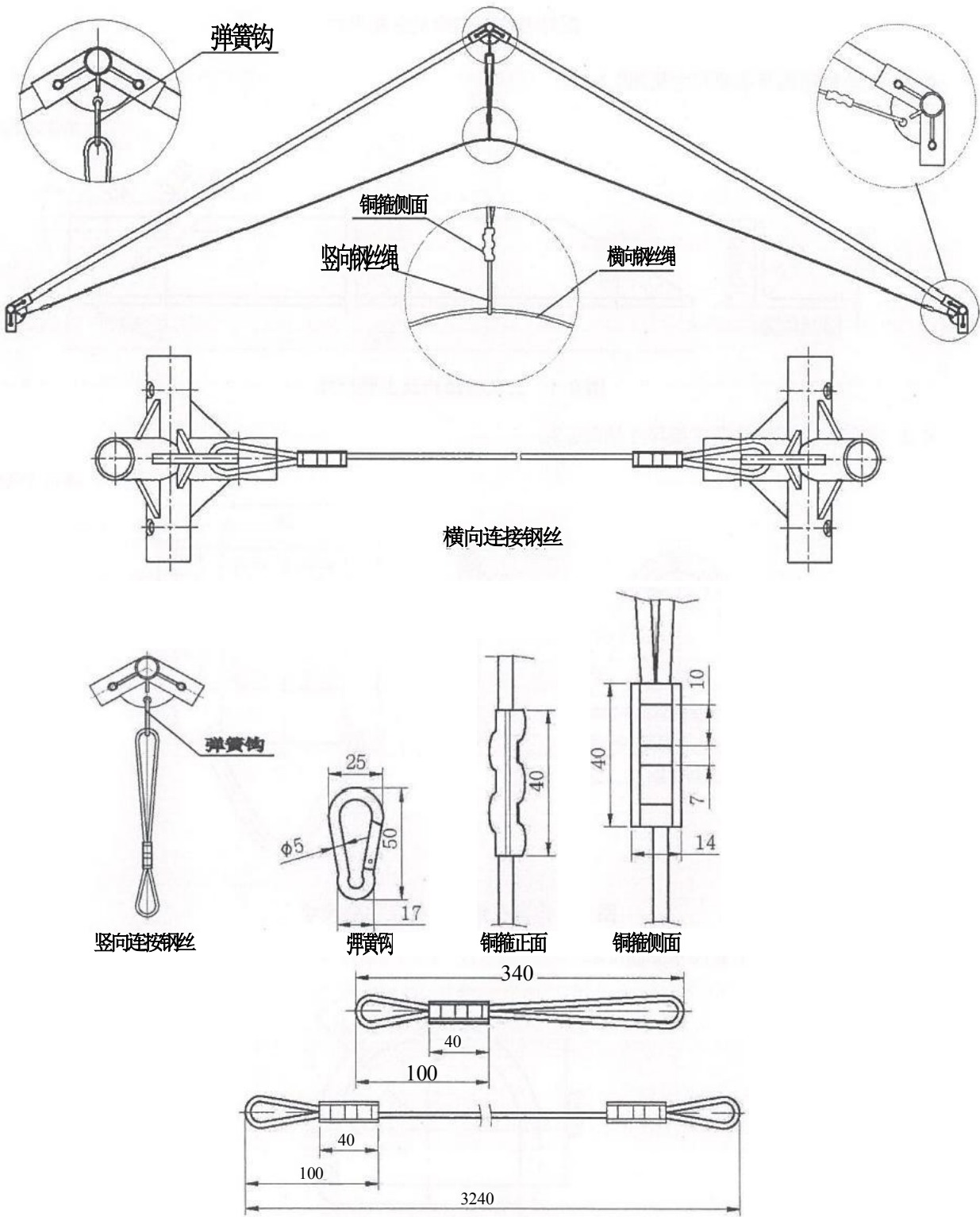
B. 8 钢丝拉绳结构及主要尺寸
