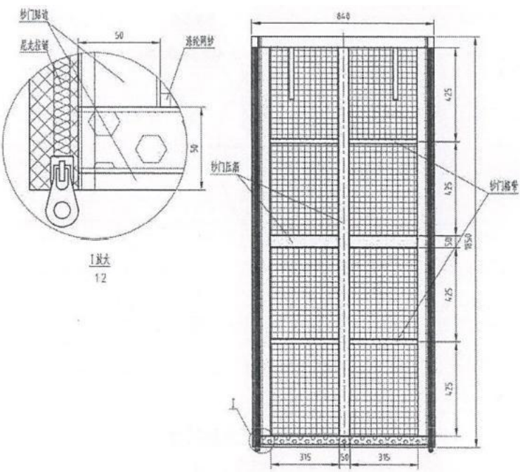
图 A.11 纱门结构及主要尺寸
