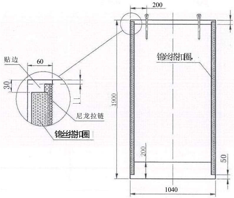
图A.10 门帘结构及主要尺寸
