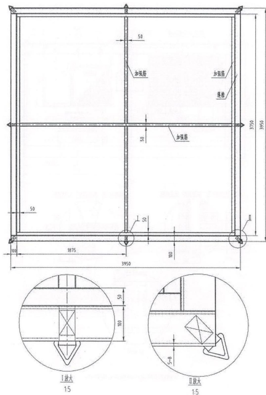
图 A.2 篷顶里结构及主要尺寸
