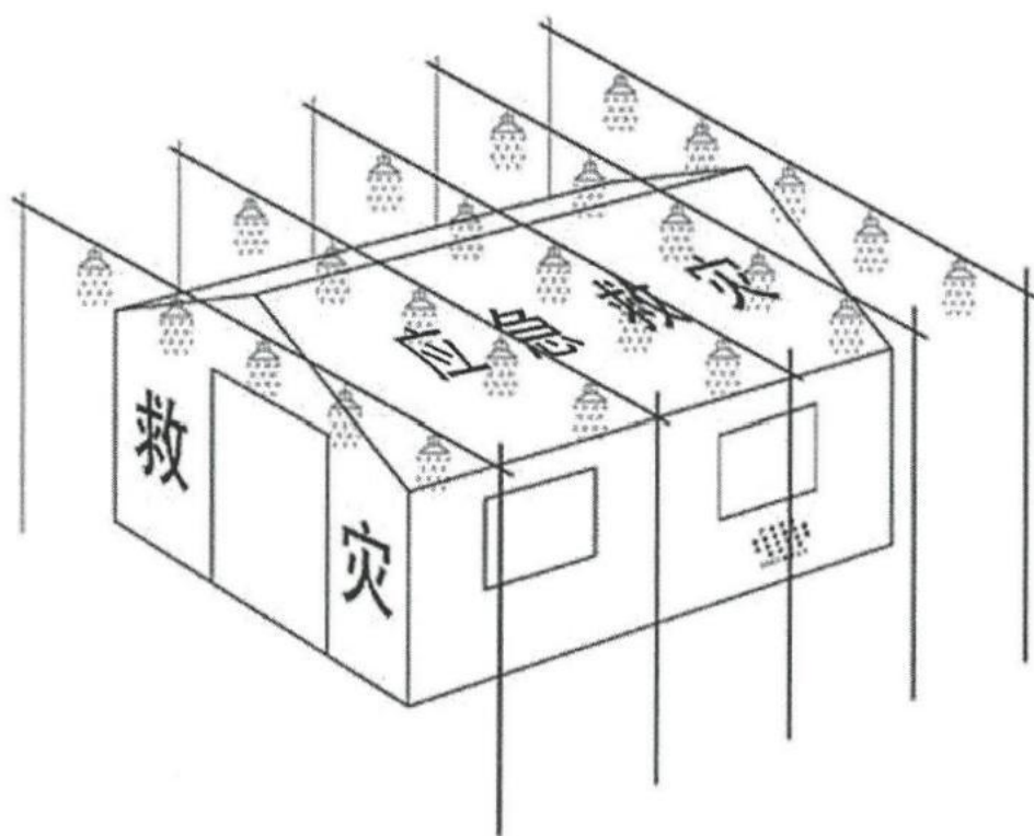
图 D.1 防雨性能试验示意图
