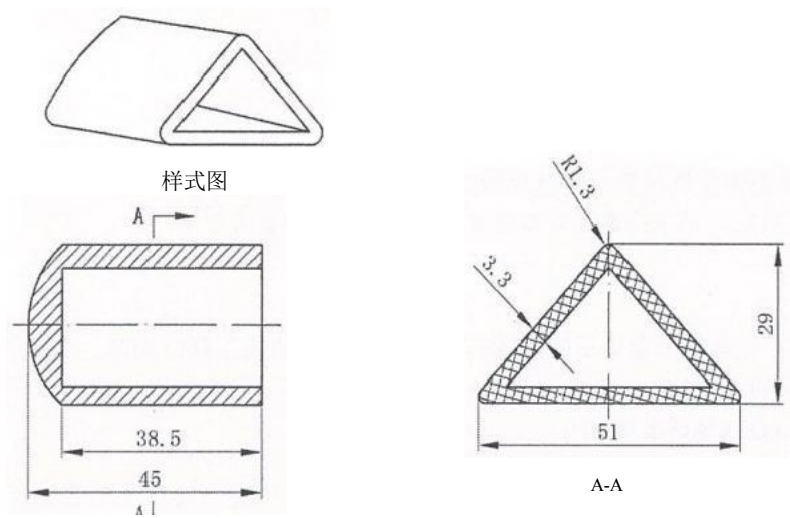
图 C. 4 橡塑桩头结构及主要尺寸
