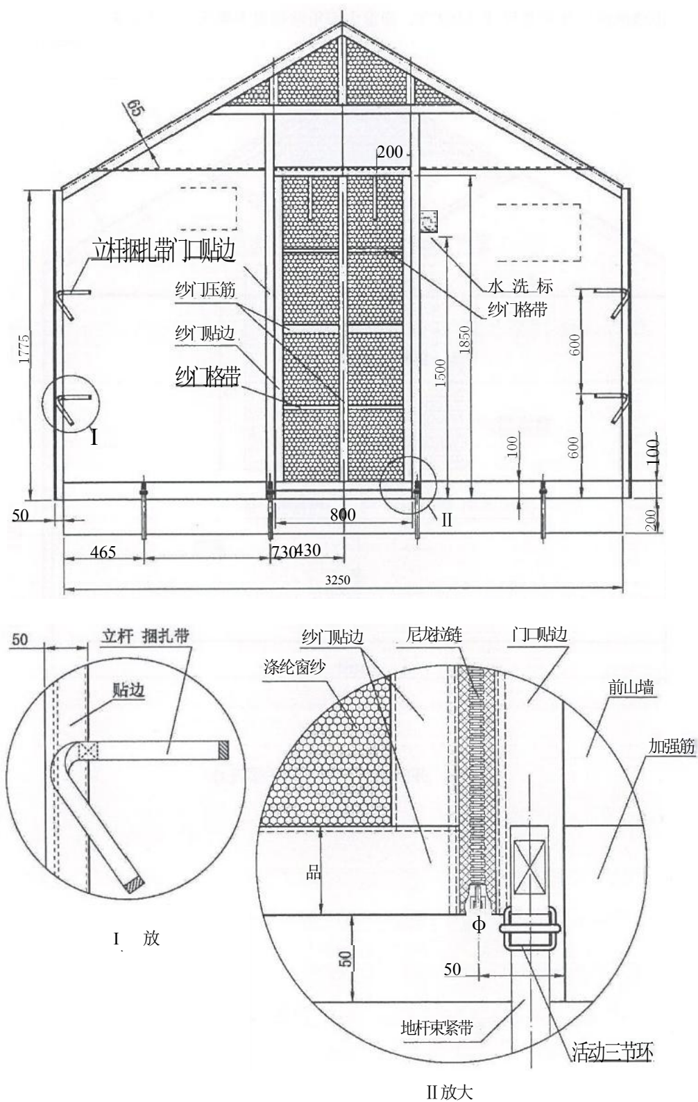
图 A.6 开门山墙里结构及主要尺寸
