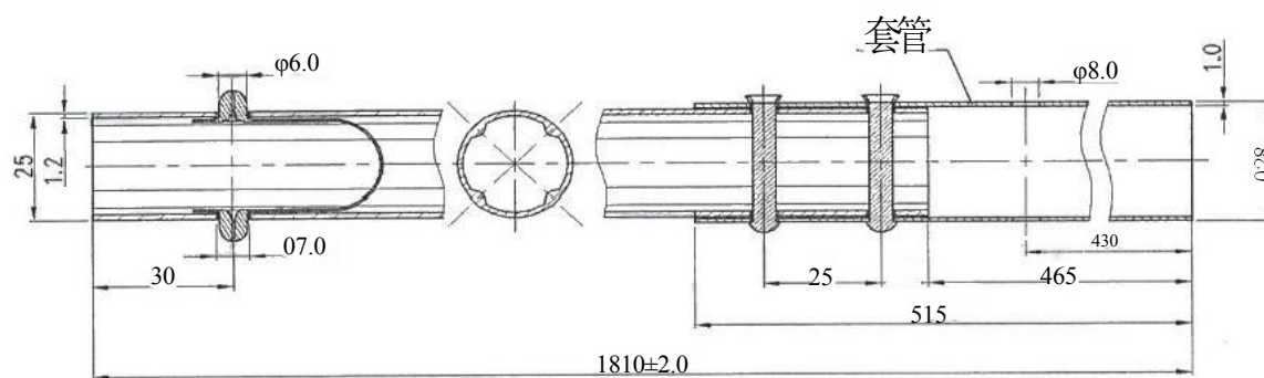
图 B.3 山墙地杆结构及主要尺寸
