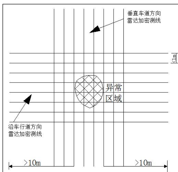
图 6-4 异常区域复测测线布置示意图
