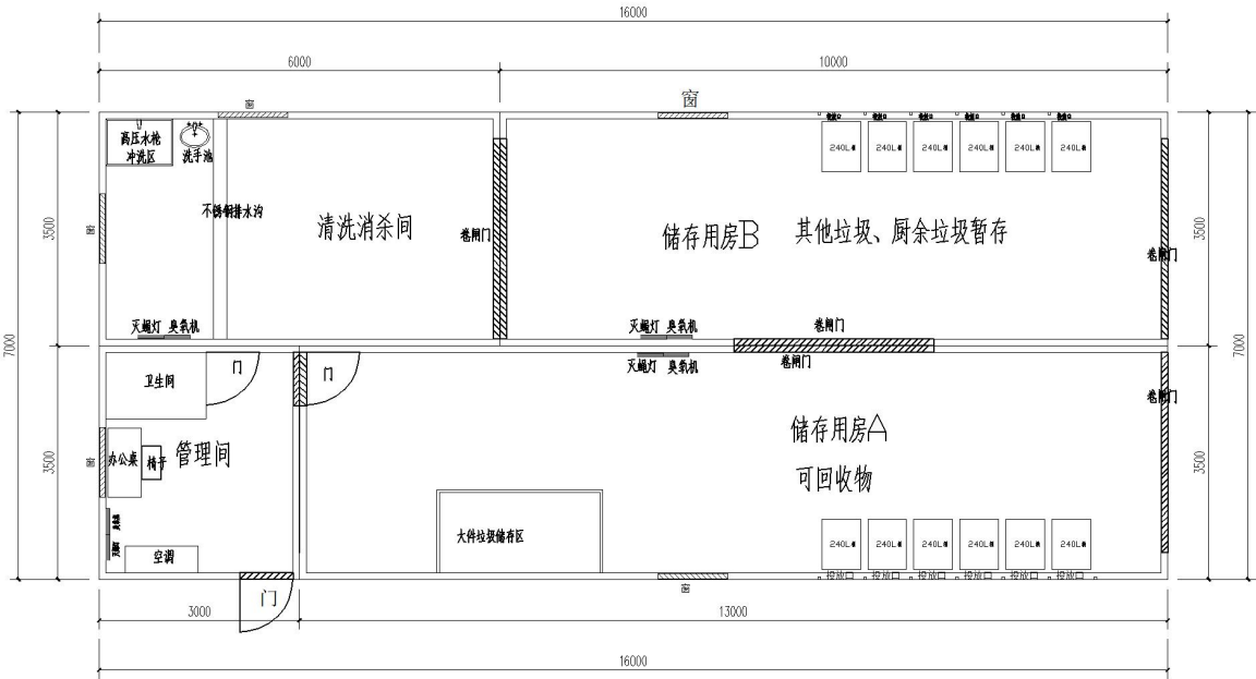
暂存点布局示例图
