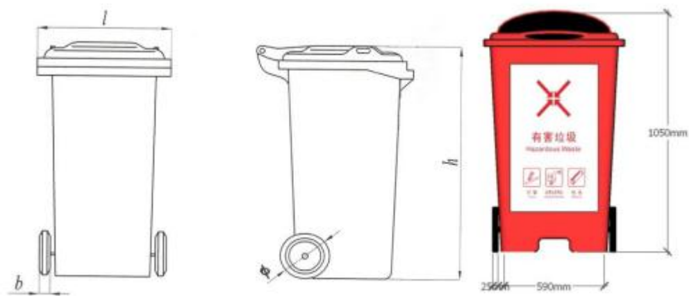
标准塑料垃圾桶（240L）外形结构
