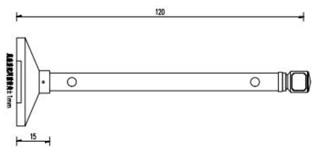
机顶主臂横断面图 1:10
