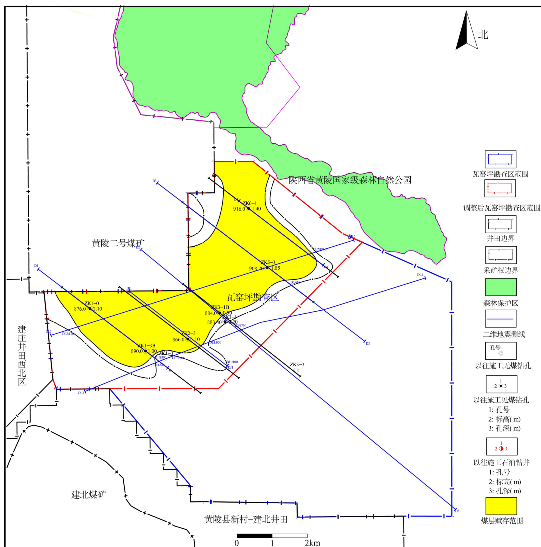
图3 煤层赋存范围示意图
