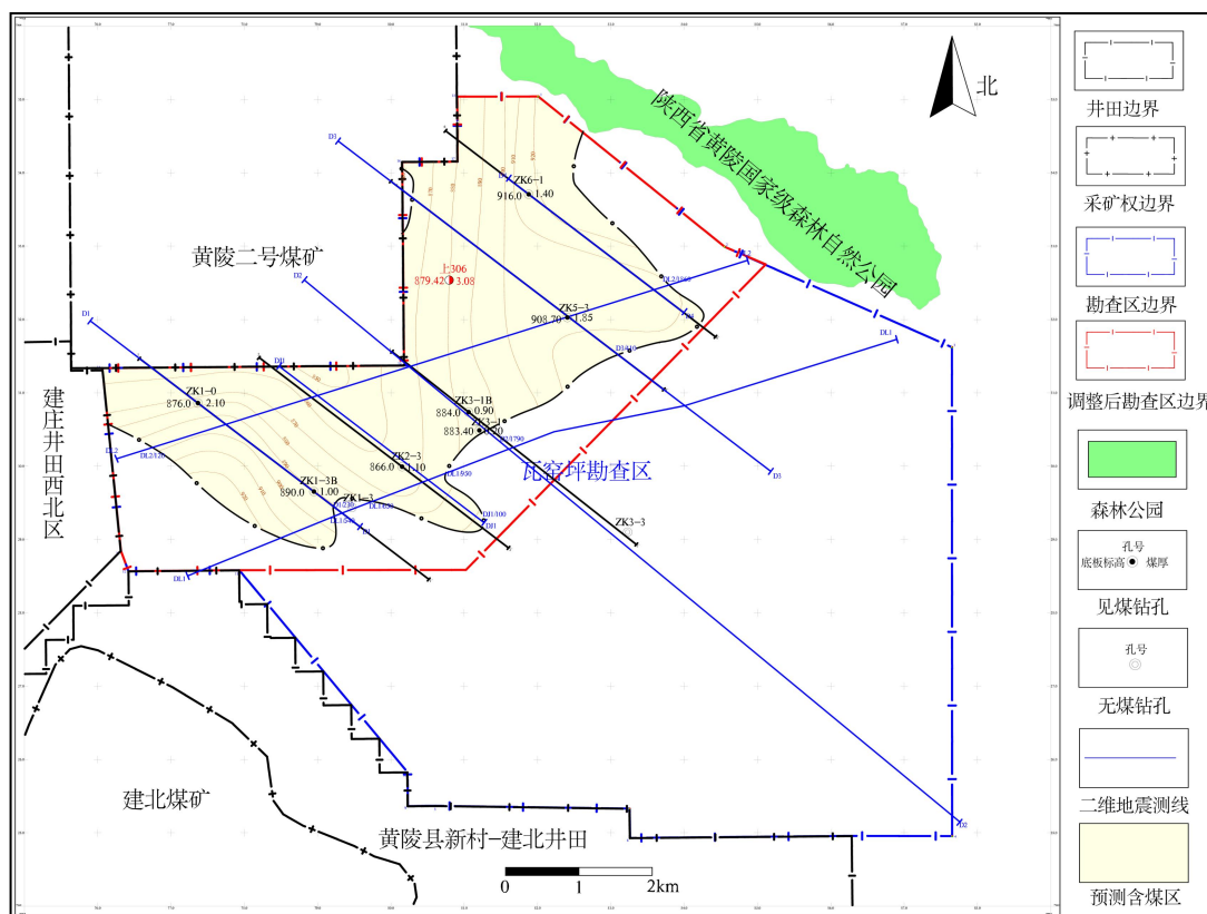
图 1 二维地震解释煤层成果图
