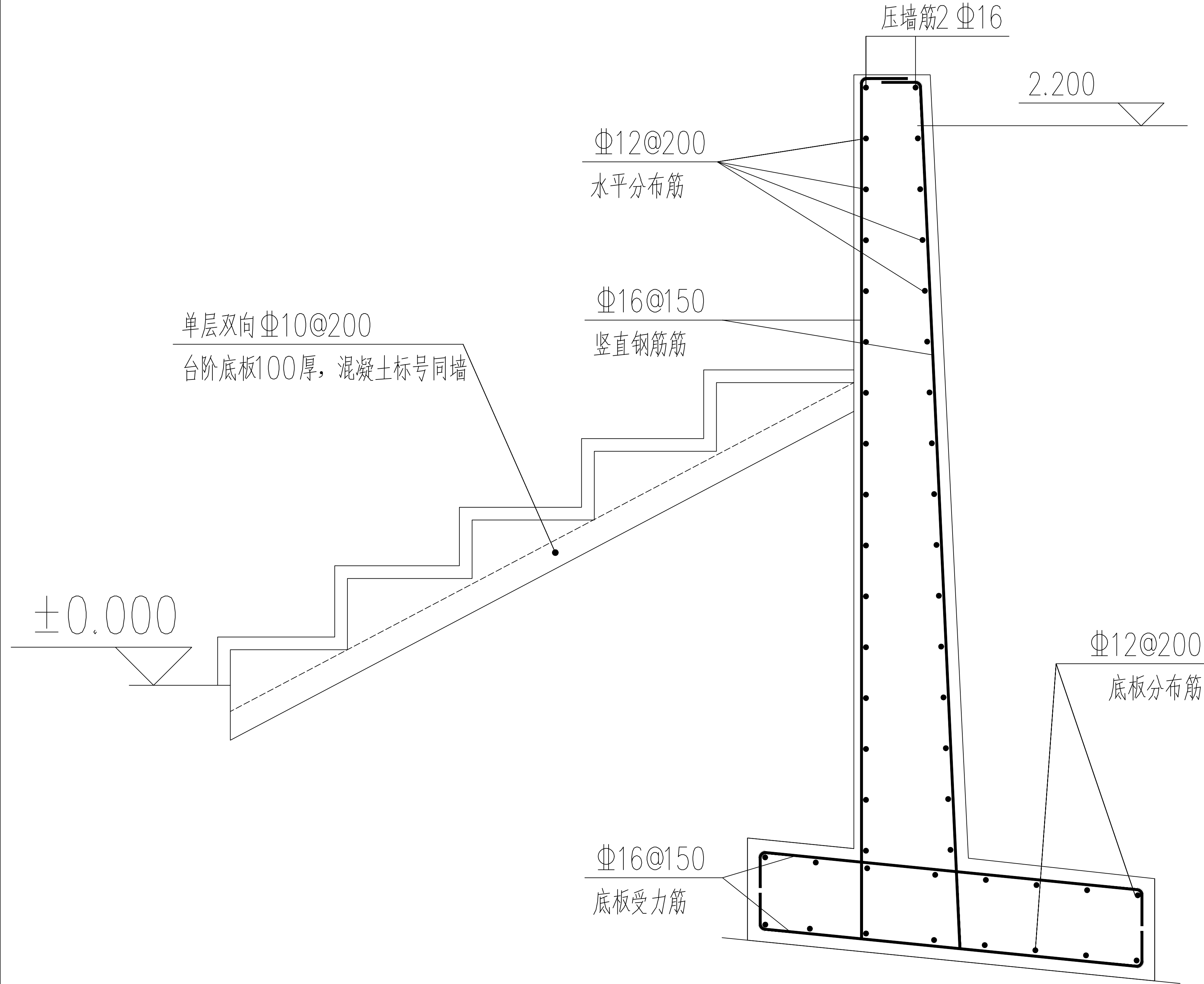
挡土墙配筋图 1:10
