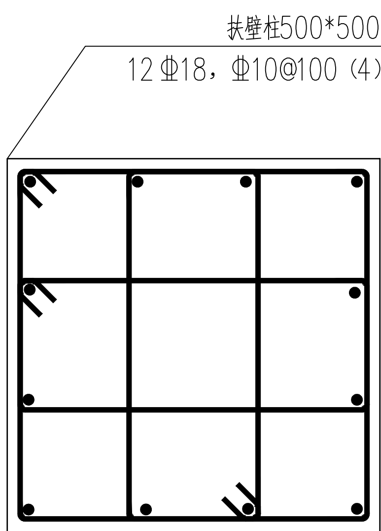
扶壁柱配筋图 1:10
