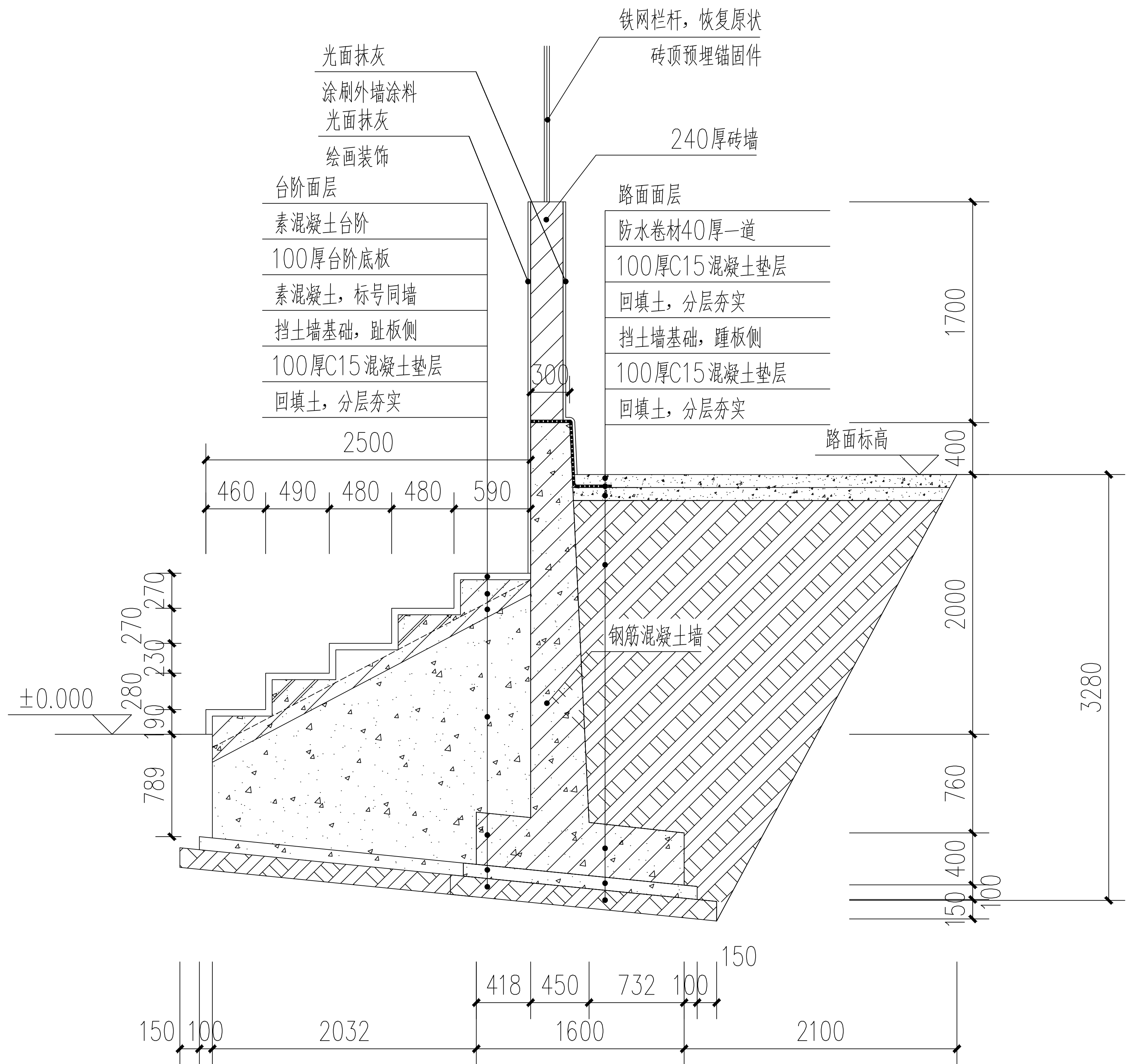
挡土墙剖面图 1:20
