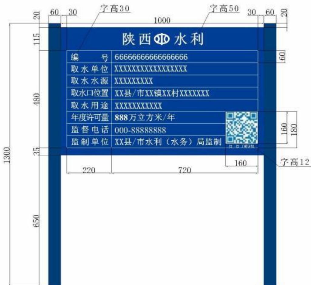
双立柱式取水口标示牌示意图
