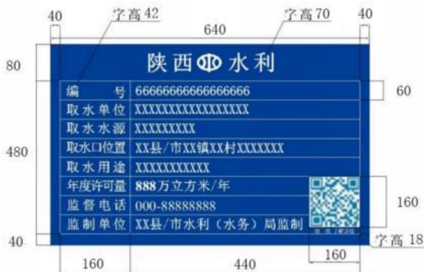
贴牌式取水口标示牌示意图
