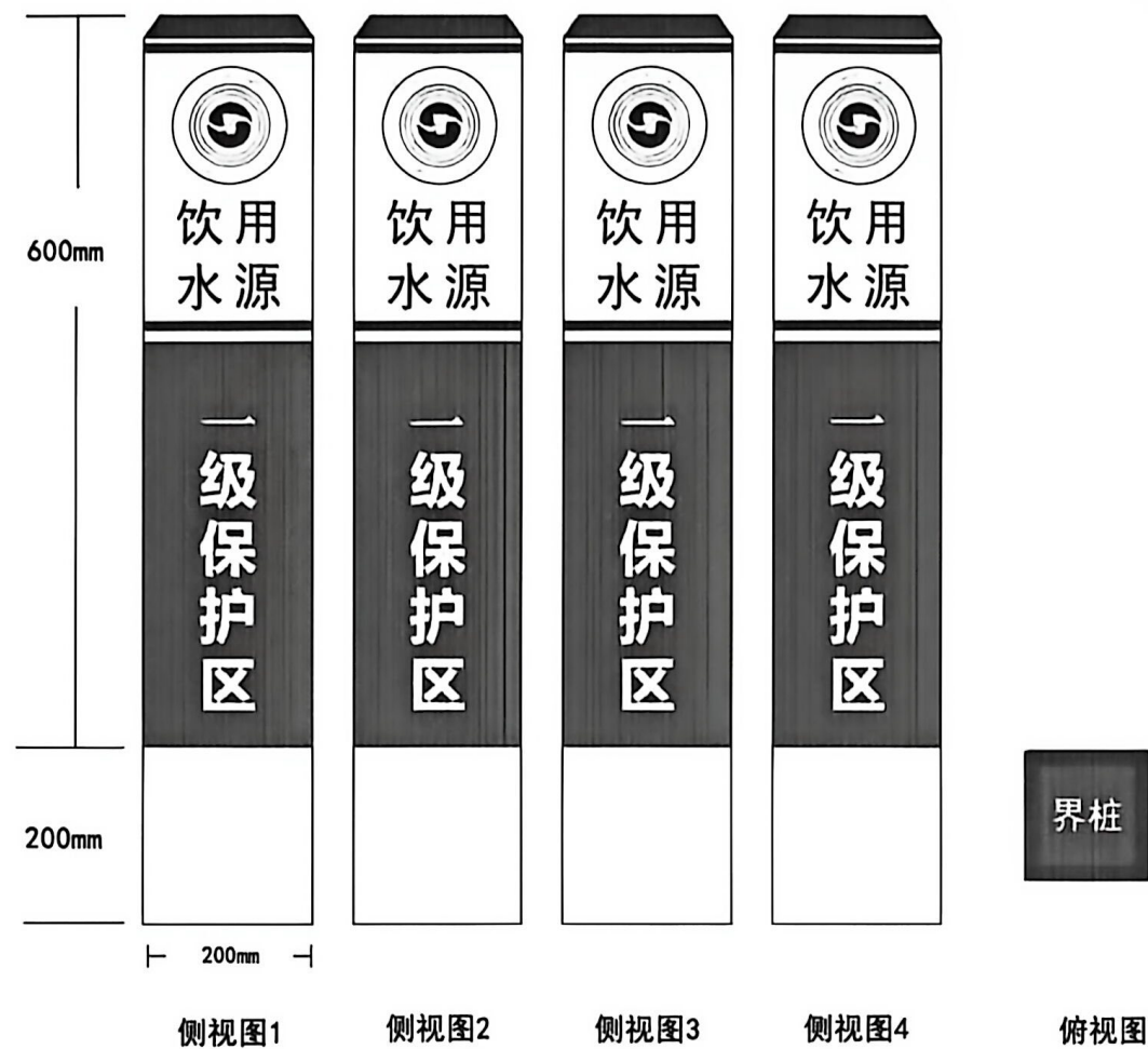
界桩示意图
