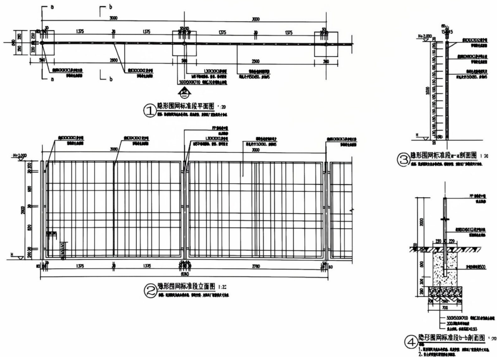
隔离防护网
