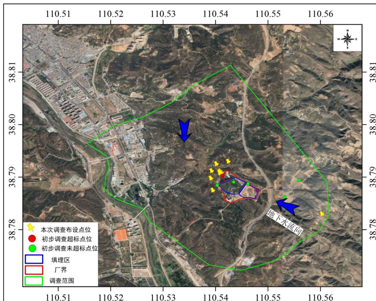
图1 神木市生活垃圾卫生填埋场地下水监测井布设图
