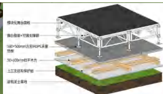
舞台结构图
