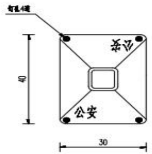
底座大样图 1:10
