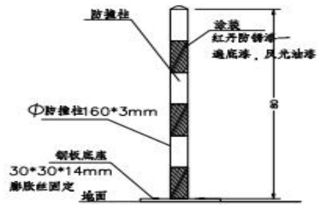
防碰柱立面安装布置图
