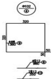
立柱帽
