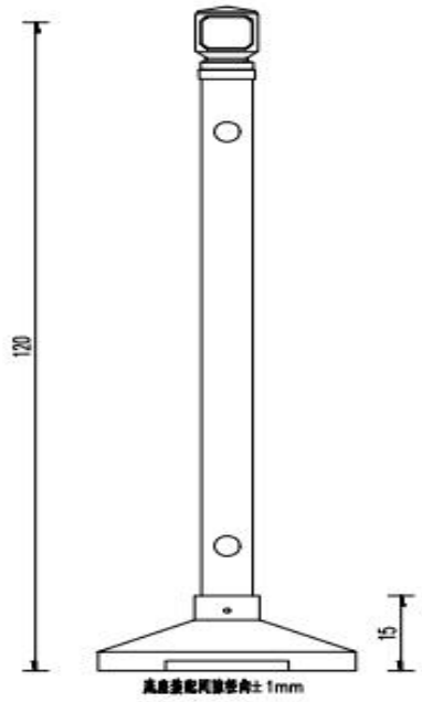
机动车隔离栏断面图 1:10
