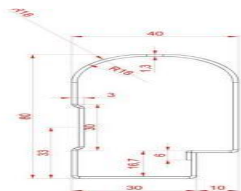
前后床厅尺寸参考图
