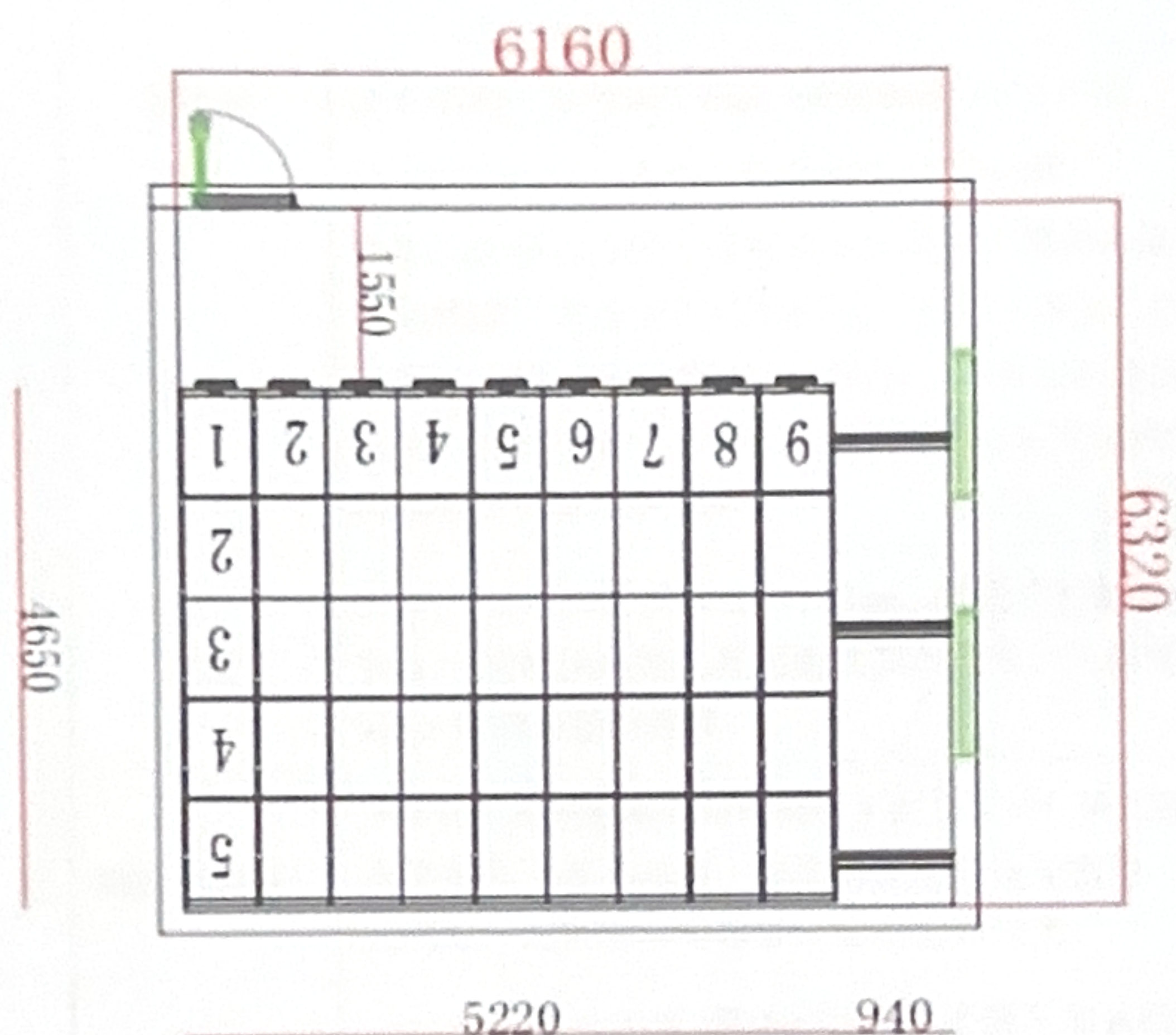
现场布置图:
